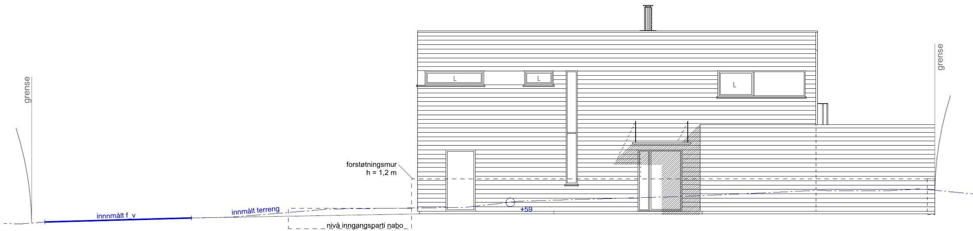
fasade NORD
